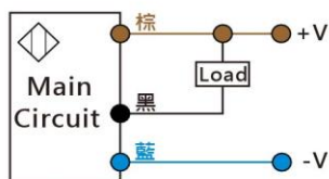
直流3線 NPN NO
