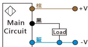
直流3線 PNP NO
