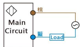
交流2線 NO
